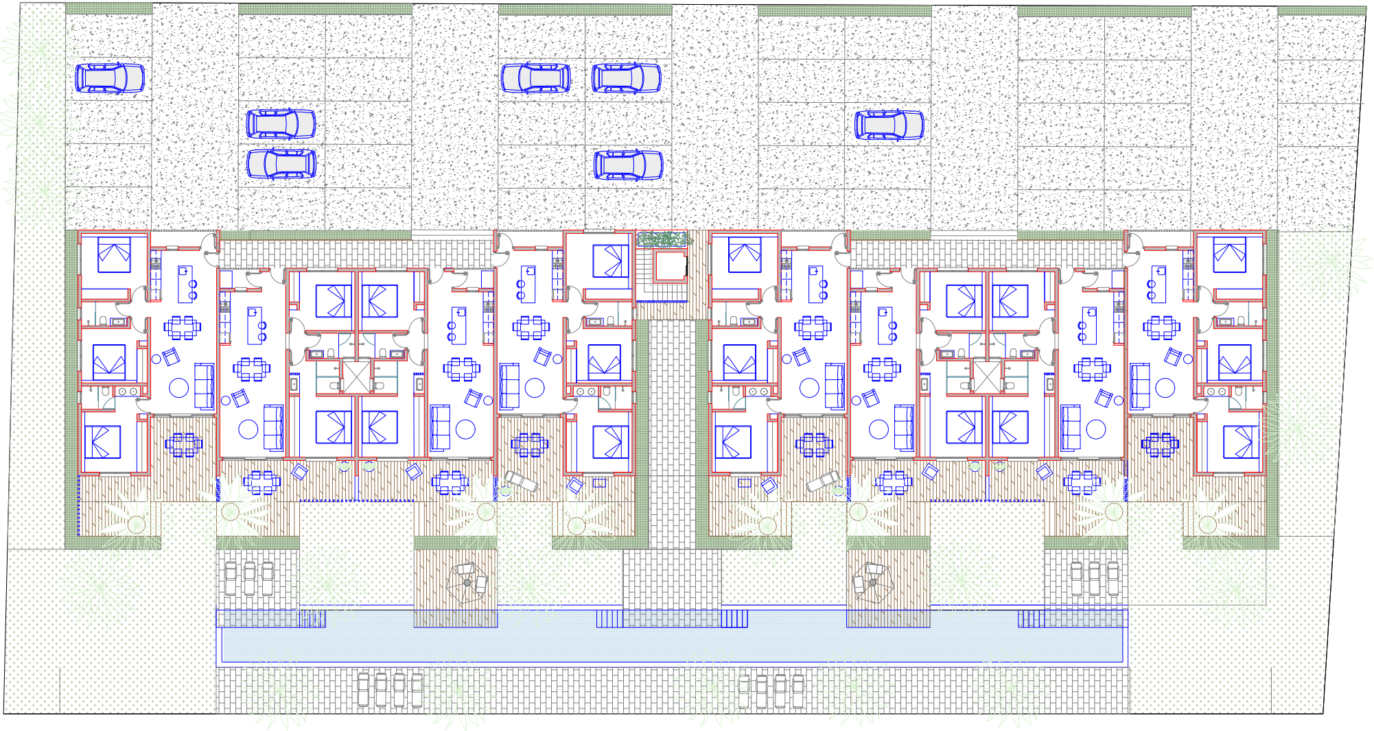
PLANTA BAJA
